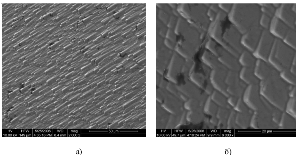
Рис. 2. Боковая поверхность непланарной кремниевой подложки: а) рельеф в виде прямоугольных ступеней; б) рельеф в виде угловых уступов
