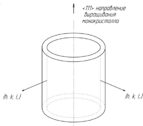
Рис. 1. Непланарная полупроводниковая монокристаллическая подложка
