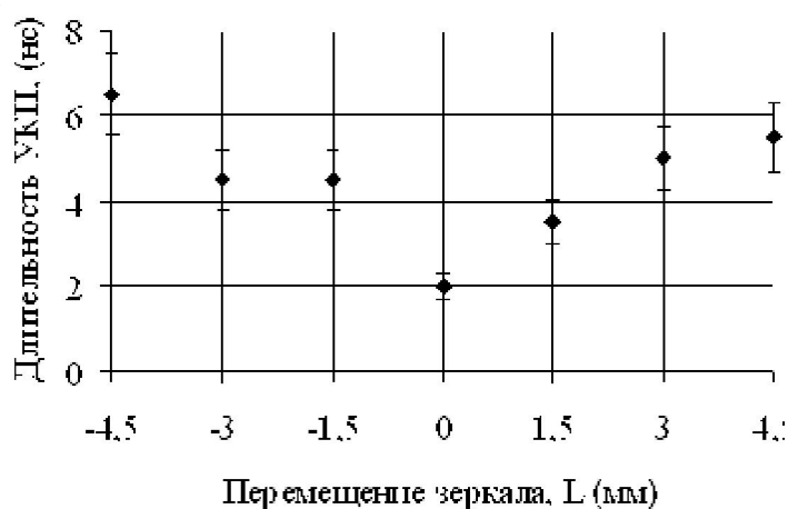
Рис. 5. График зависимости длительности одного импульса из цуга УКИ \tau_n (нс) от перемещения выходного зеркала резонатора \Delta L (мм) в режиме регенеративного усиления
