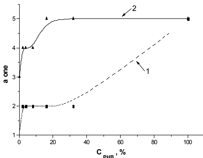
Рис. 2. Зависимость грибостойкости ПЭНП/ПГБ-пленок (в баллах) от содержания ПГБ (%): 1 – для исходных и 2 – для фотоиницированных в течение 600 часов
