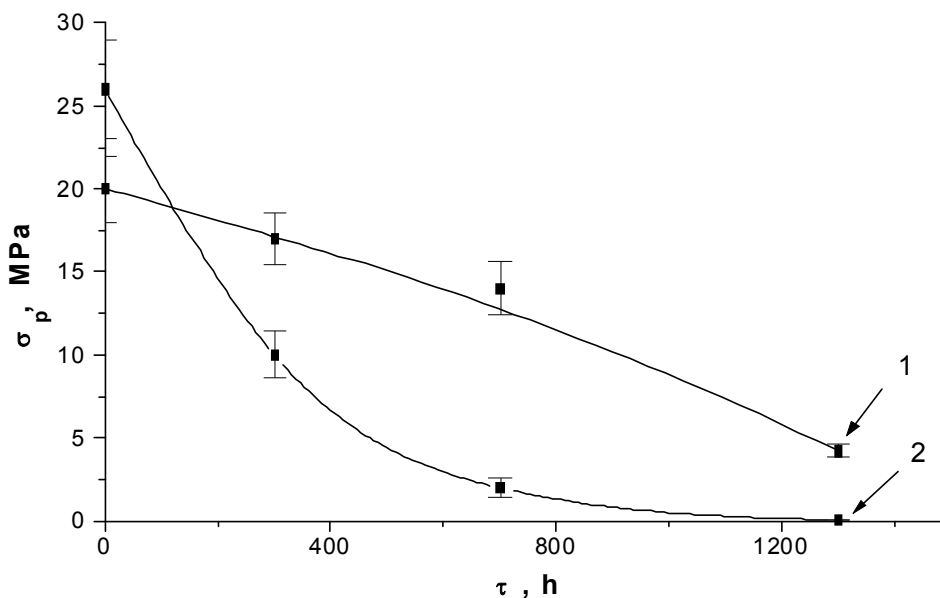
Рис. 1. Зависимость разрушающего напряжения ( \sigma_p , МПа – МПа) при растяжении пленок из ПЭНП (1) и из смеси ПЭНП (92 % масс.) и ПГБ (8 % масс.) (2) от времени старения ( \tau , h – час.)
